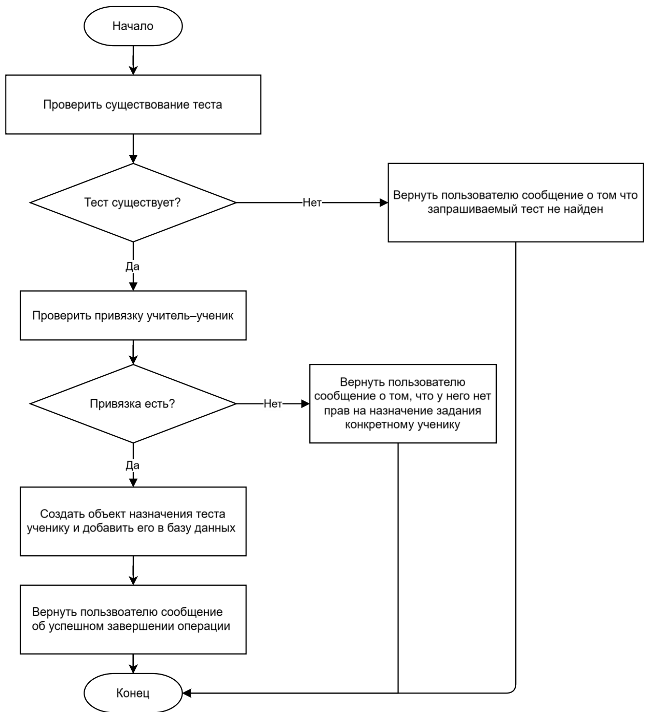
Рисунок 3.7 – Схема алгоритма назначения теста ученику
